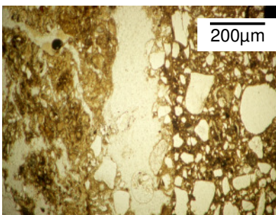
Dünnschliff-Aufnahme aus einer Dichtungsfuge, die mit herkömmlichen Tonkugeln verfüllt wurde. Unvollständige Quellung und mangelnder Randschluss durch den Einfluss von ölhaltigen Stauwässern (links: Tonpellets, rechts: Geschiebemergel)
