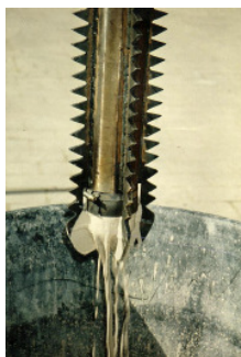
Bohrloch-Fräse mit Dichtmasse
