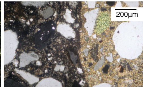
Dünnschliffaufnahme aus dem Dichtungsfugenbereich nach einer Bohrlochplombierung mit optimierten Dichtmassen, die einen vollständigen Randschluss zur Basisdichtung gewährleisten (links: Dichtmasse, rechts: Geschiebemergel)
