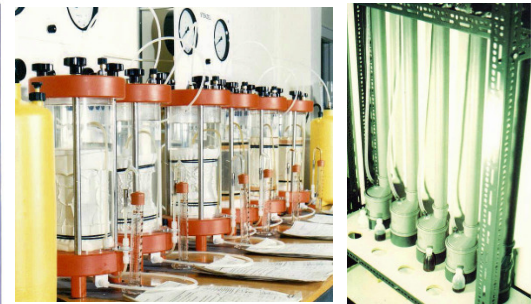
Prüfung und Optimierung der Durchlässigkeits- und Verpresseigenschaften verschiedener Dichtmassen
